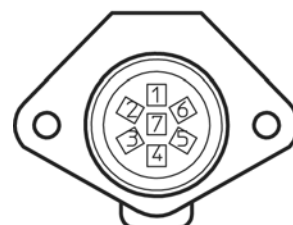
ISO 3731 : 24S (Vue arrière)
